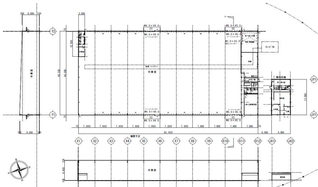
③工場立面図
