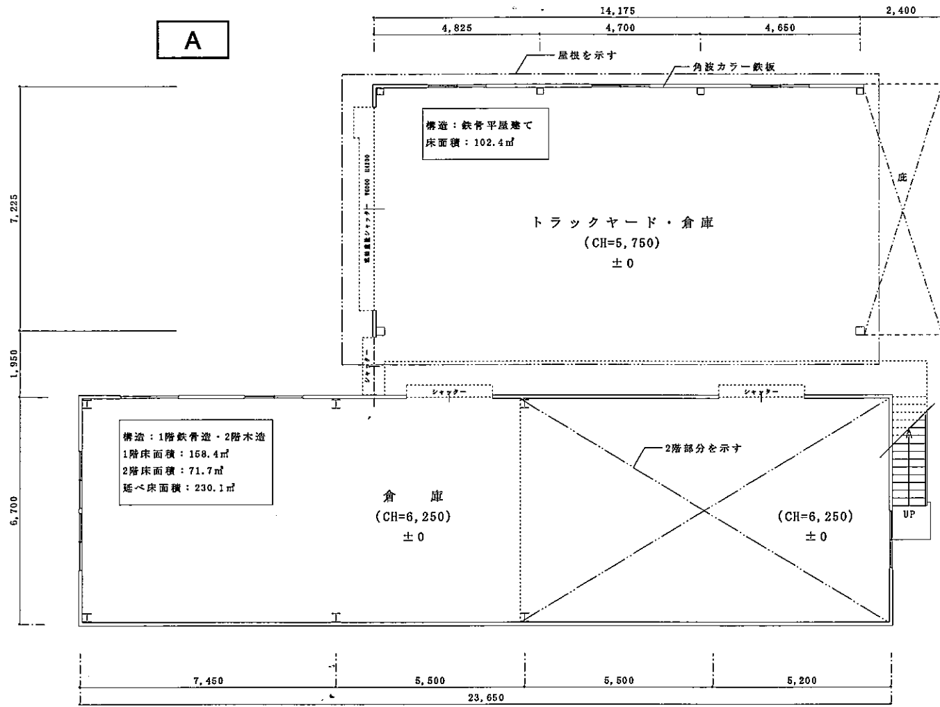
1階平面図 1/100
