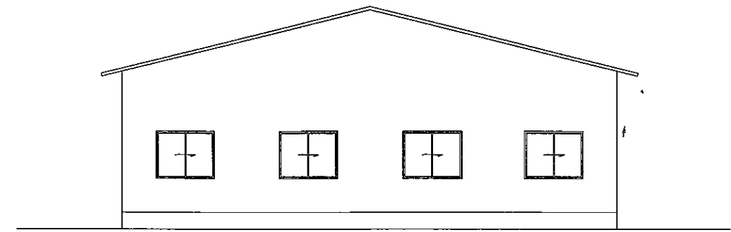
北側立面図 1/100
