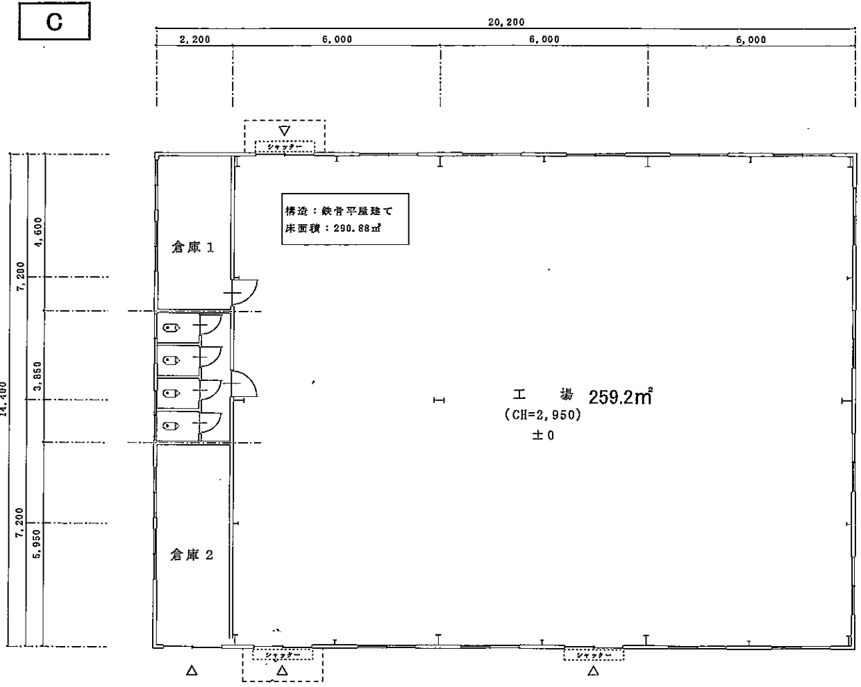
1階平面図 1/100
