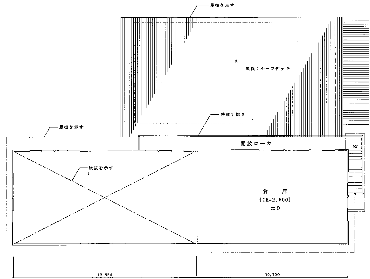
2階平面図 1/100
