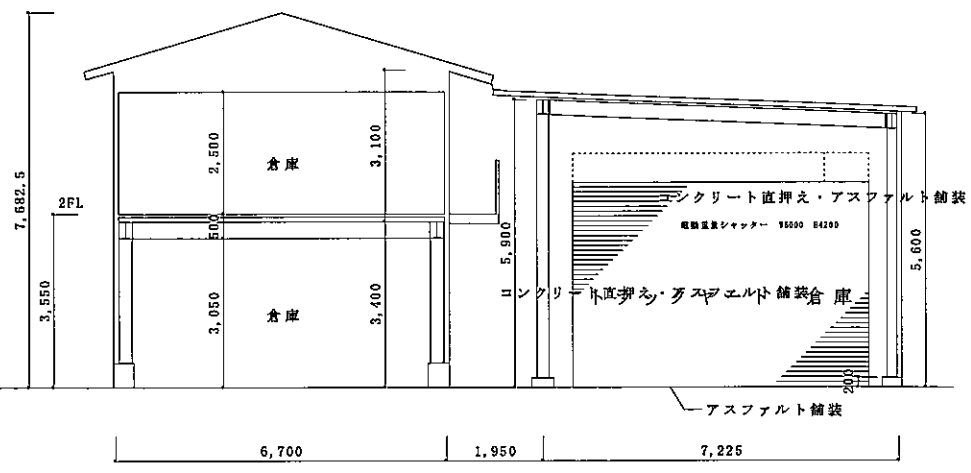
断面図 1/100
