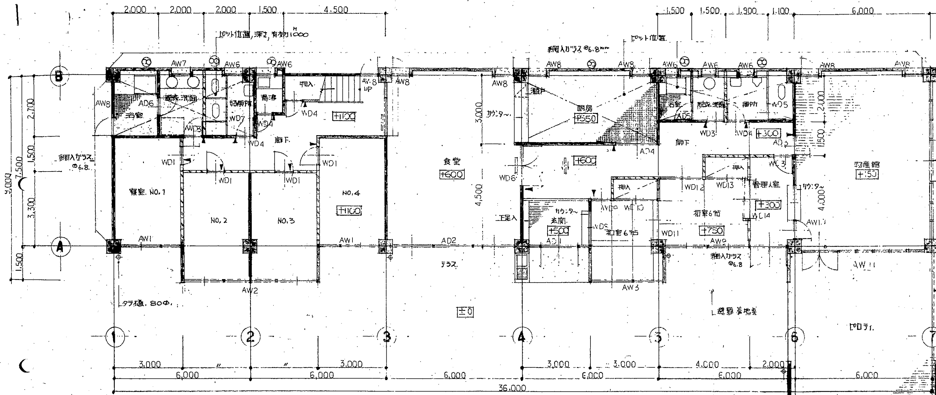
1階平面図 1:100
