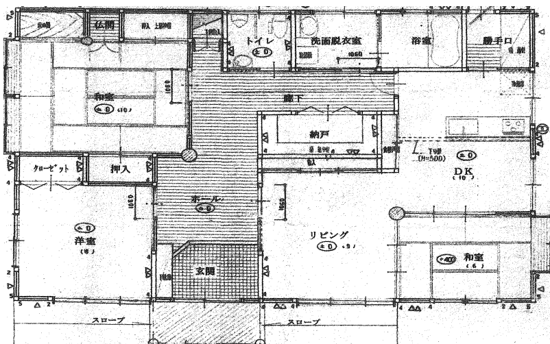
平面図
